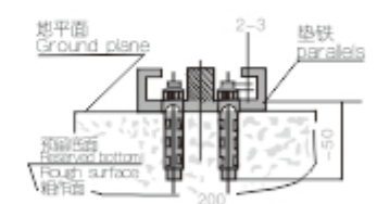
地面式轨道组断面图 Ground track group section
