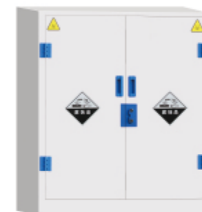
MY-IC-11 H1120*W1090*D460mm
